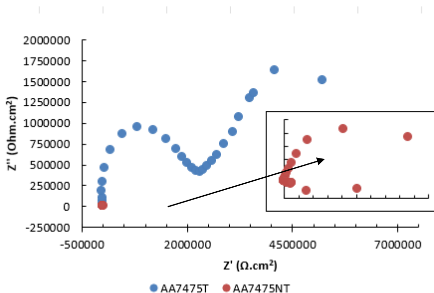
Figura 10: Diagrama de Nyquist da liga AA7475 tratada e não tratada em NaCl 3,5% (m/v).
